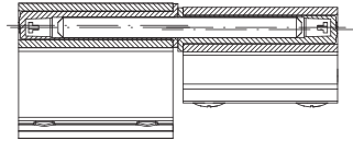
Presek B-B
