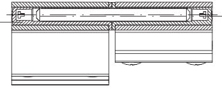
Presek A-A
