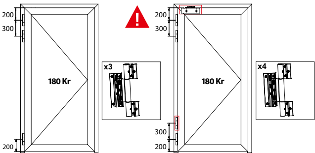
Максимальный вес дверной створки при использовании 3х петель „Rollenband AT“
